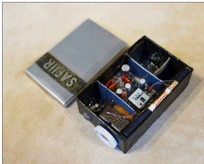
1973.a. valminud väike taskuraadio
