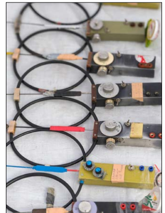
80 m laineala peilingaatorid. Fotod Leedu ARDF
